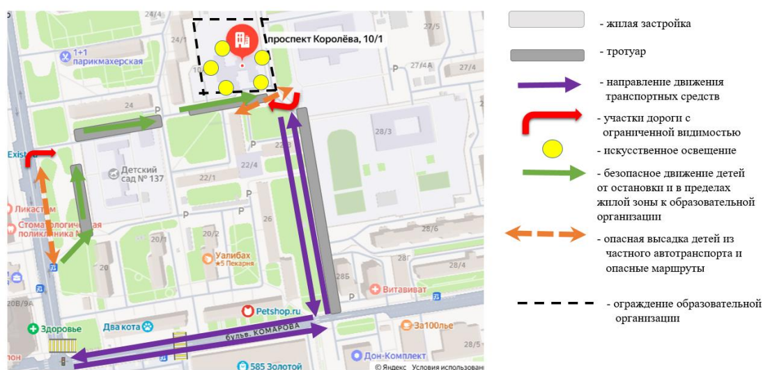
Организация дорожного движения в непосредственной близости от МБДОУ № 137 с размещением соответствующих технических средств организации дорожного движения, маршруты движения детей и расположение парковочных мест
